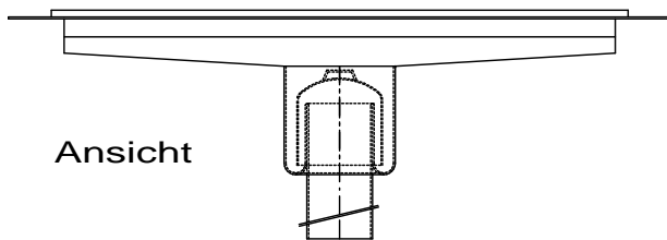
Duschenrinne mit Sifon vertikal
