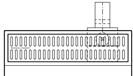
Grundriss
